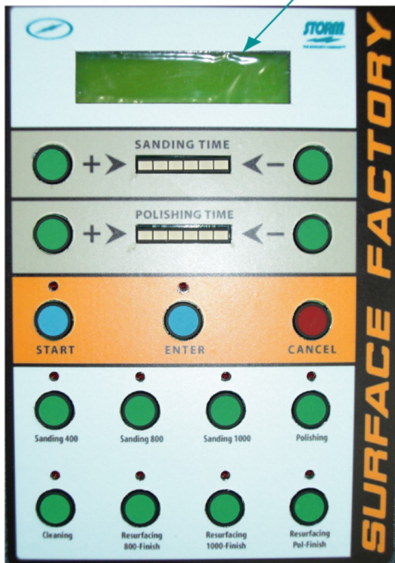
操作パネル
